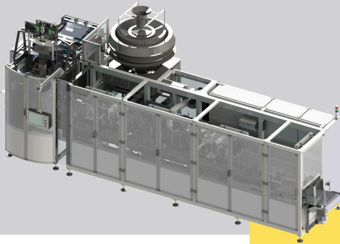
Peseuse multi-têtes
